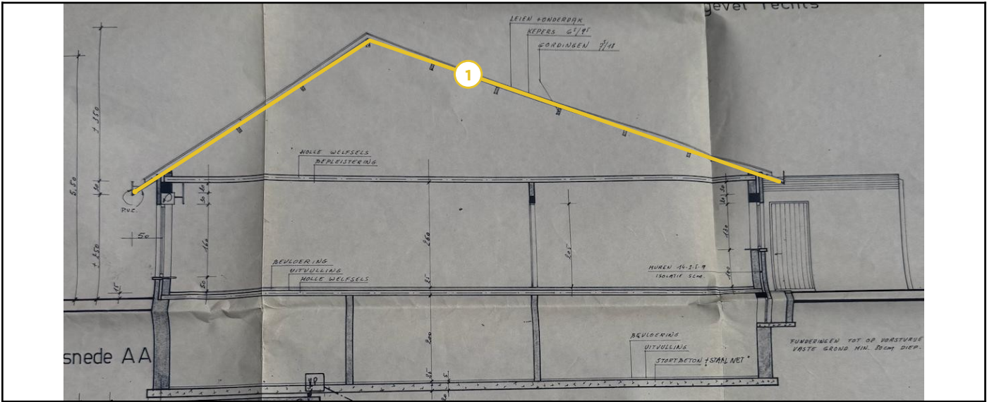
Legende van plan 1.3: Doorsnede
