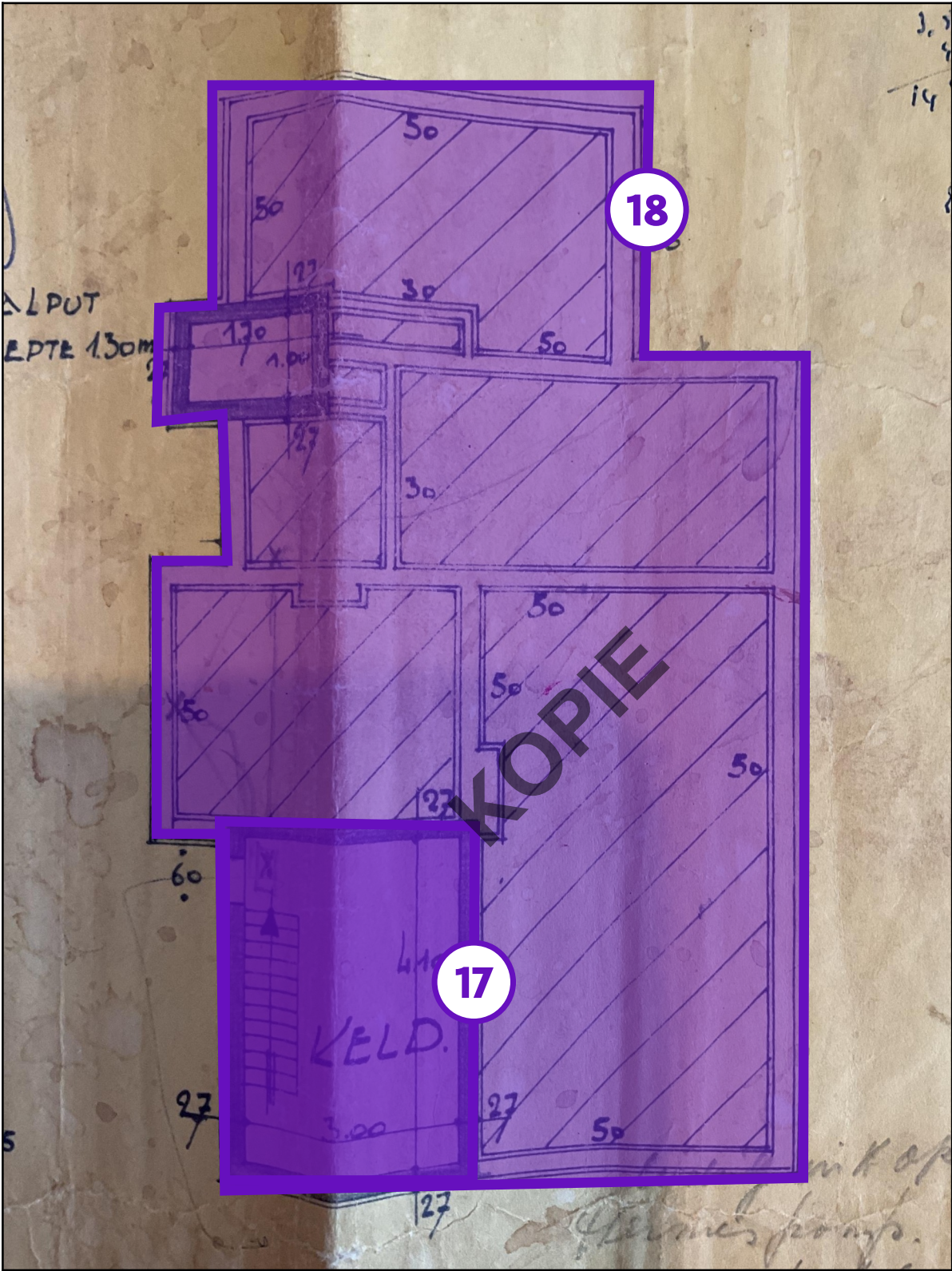
Legende van plan 1.3: Plan van de kelder
