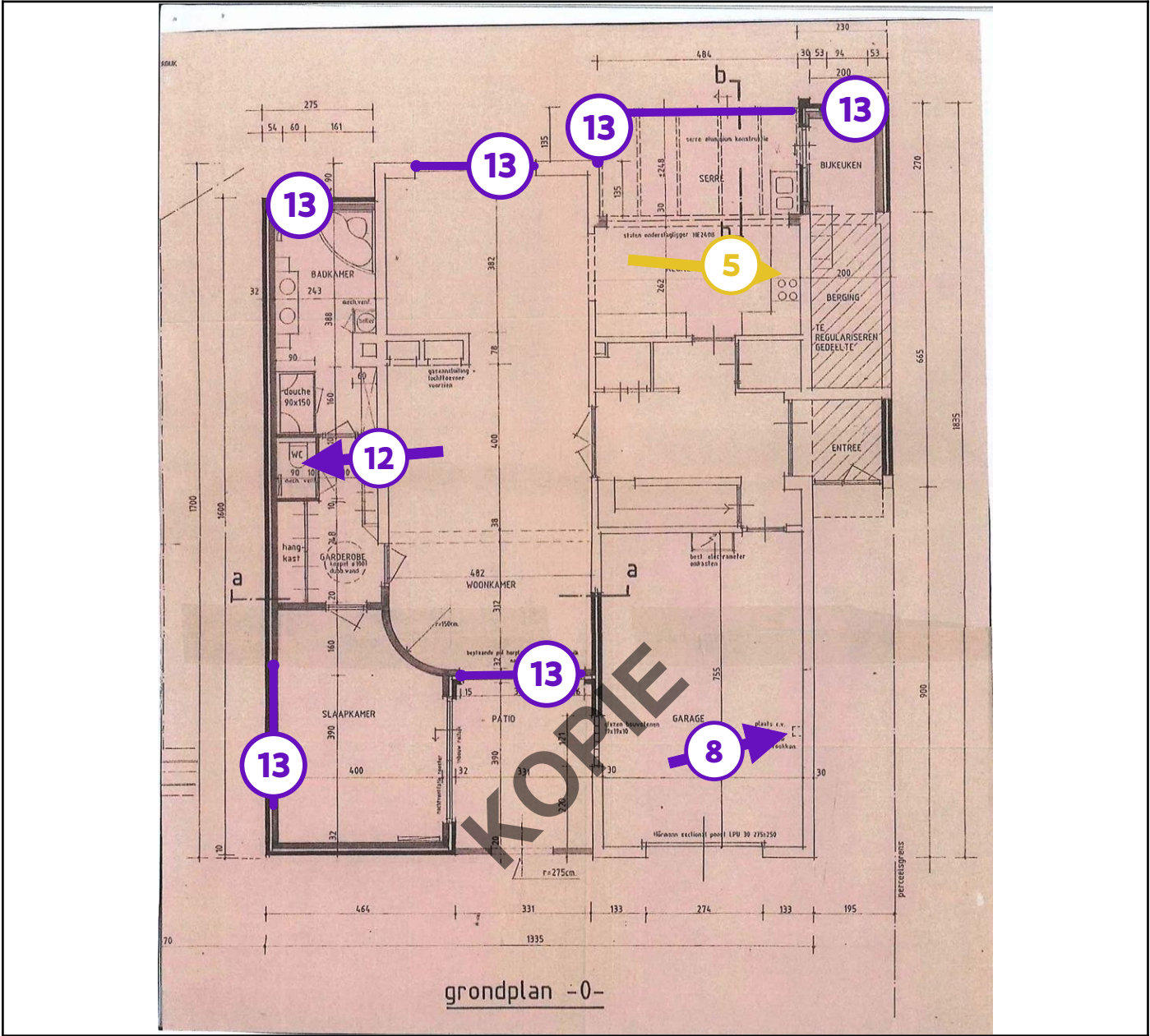
Legende van plan 1.4: gelijkvloers
