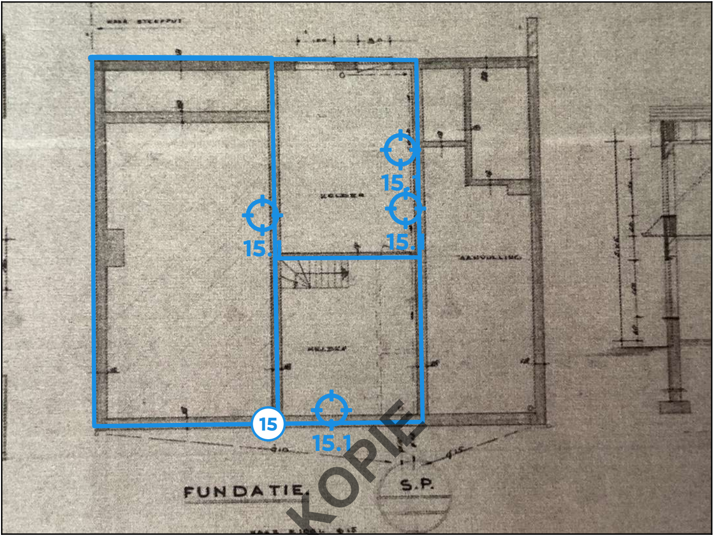
Legende van plan 1.1: Plan van de kelder
