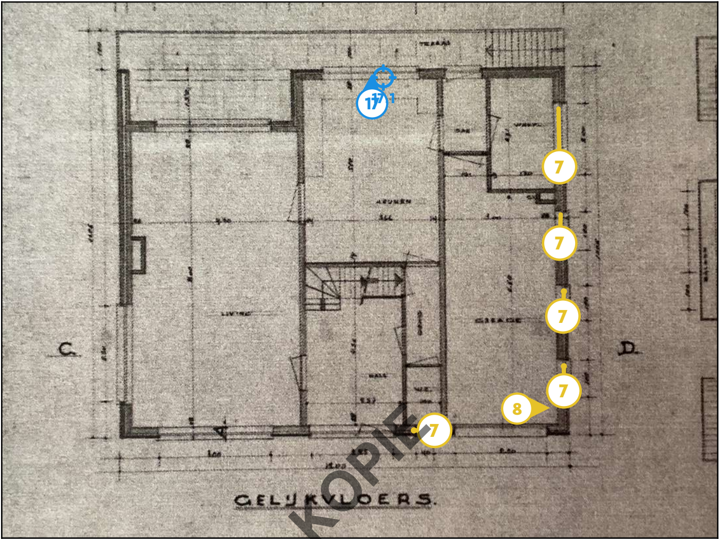
Legende van plan 1.7: Plan van het gelijkvloers
