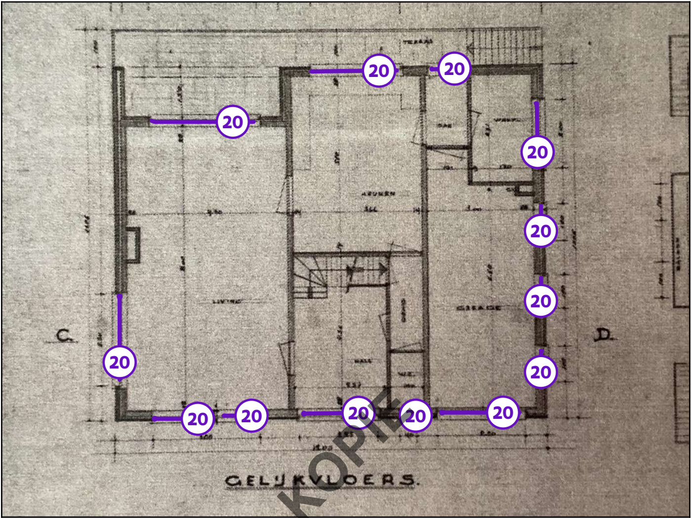
Legende van plan 1.9: Plan van het gelijkvloers
