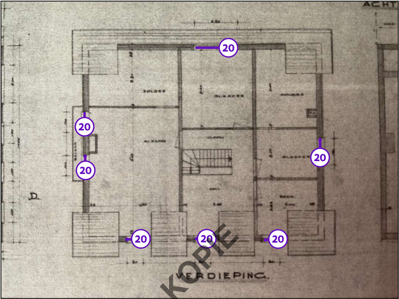
Legende van plan 1.15: Plan van de eerste verdieping
