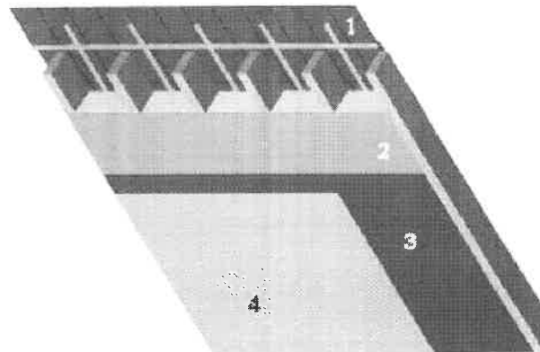
1. Onderdak | 2. Isolatie | 3. Damperscherm | 4. binnenafwerking
