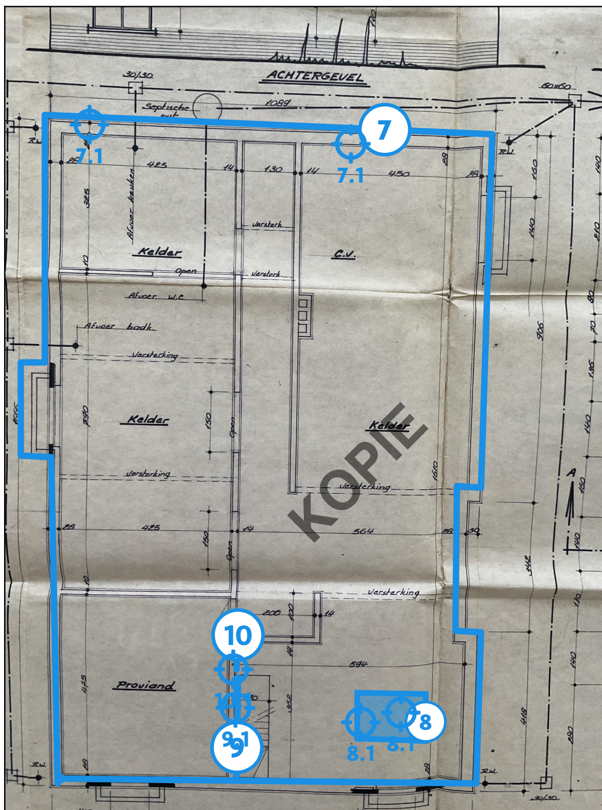
Legende van plan 1.1: Plan van de kelder
