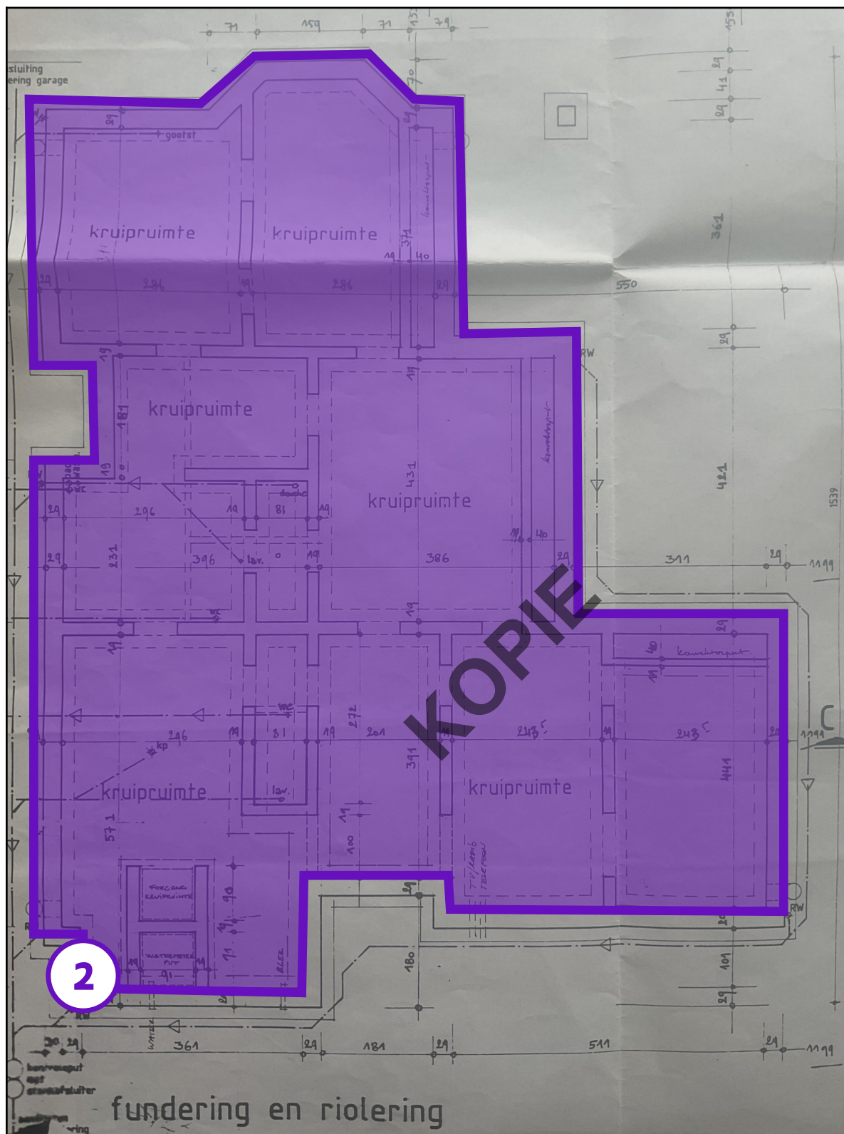
Legende van plan 1.1: Plan van de funderingen en de riolering
