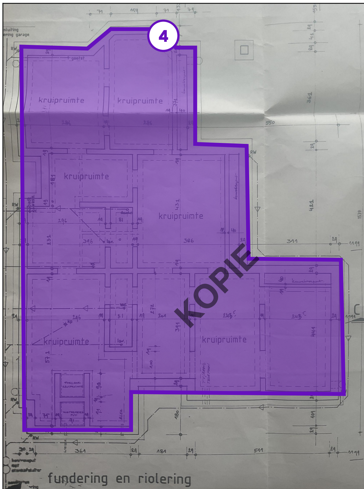
Legende van plan 1.2: Plan van de funderingen en de riolering
