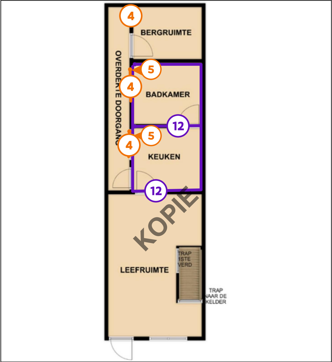
Legende van plan 1.2: Plan van het gelijkvloers
